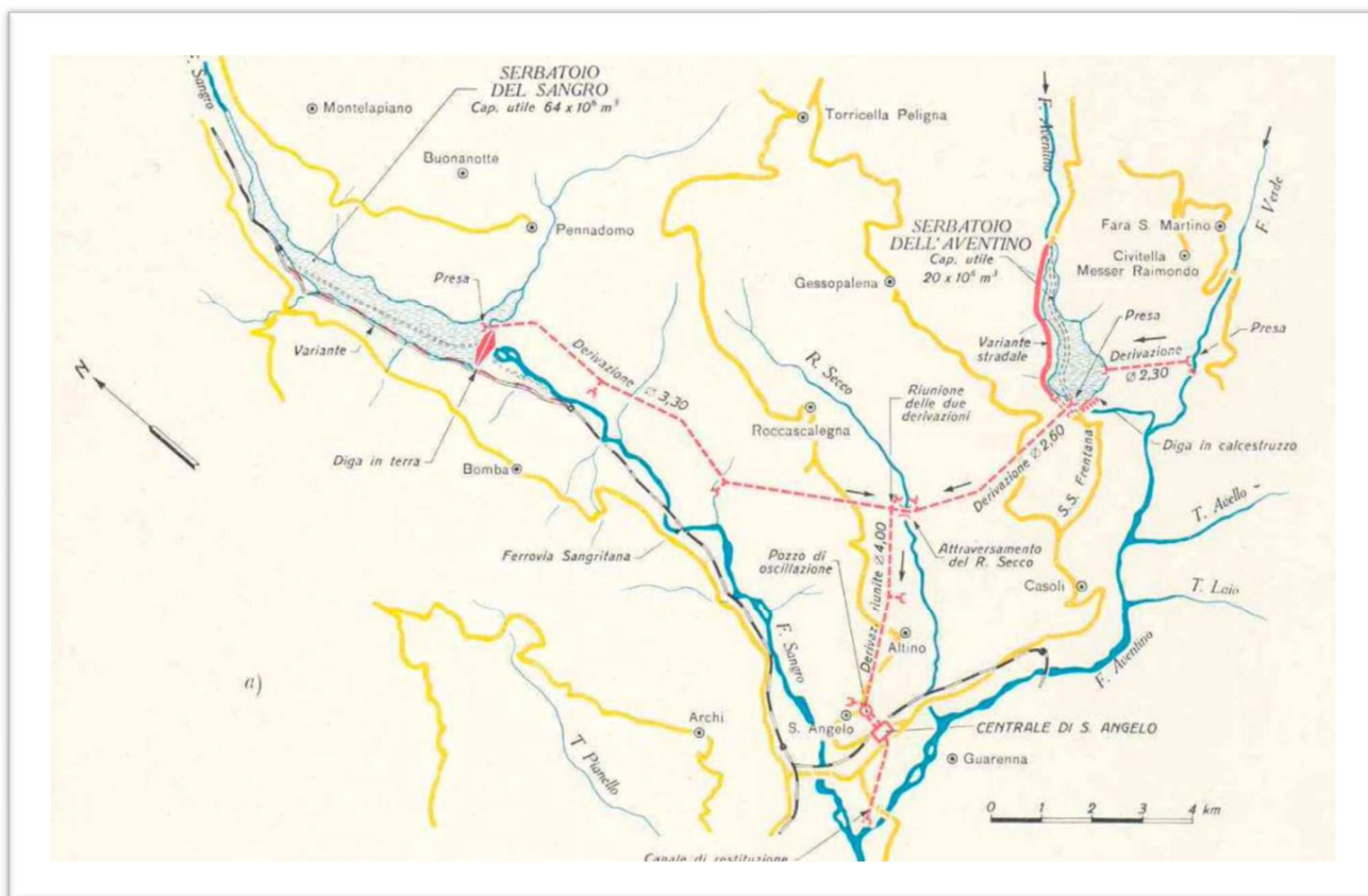
Figura 4: Dettaglio planimetrico dell'impianto idroelettrico "Sant'Angelo"
